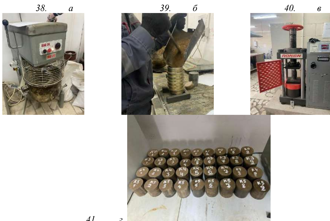
Рисунок 1. Проведение лабораторных испытаний: а – смешивание смеси; б – подготовка образца; в – испытание образцов на прочность; г – готовые образцы. Методика проведения лабораторных испытаний:
