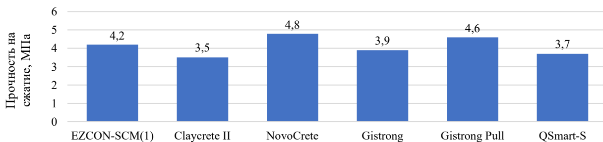
Рисунок 2. Результаты испытаний прочности на сжатие на 28 сутки
