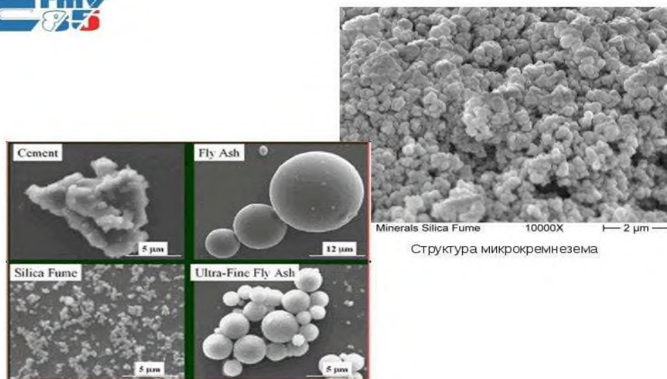
Сурет-3. Портландцементтің, күлдің және микрокремнеземның бөлшектерінің өлшемдерін салыстыру
