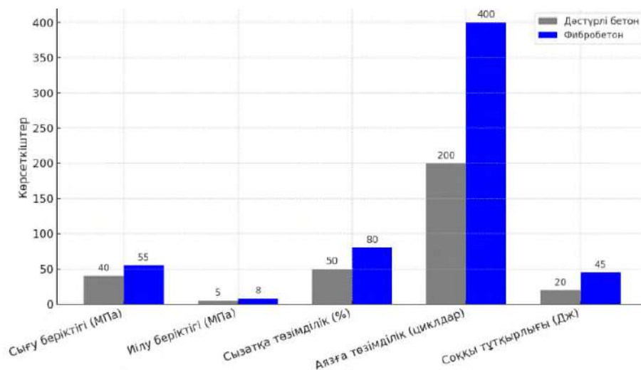
3 сурет – Дәстүрлі бетон мен фибробетонның салыстыруы
