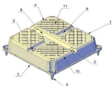
Рисунок 1. Общий вид пустотообразователя одиночной формы
