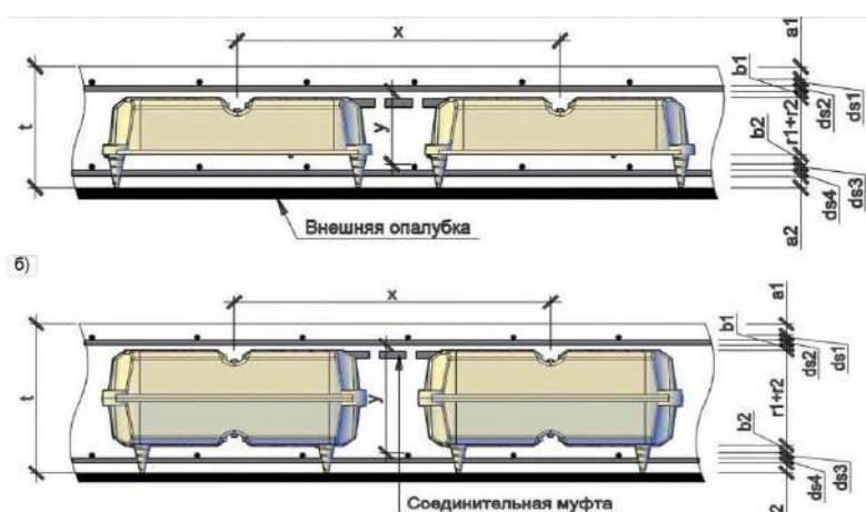
Рисунок 4. Схема возможного размещения пустообразователей и армирования перекрытия:
