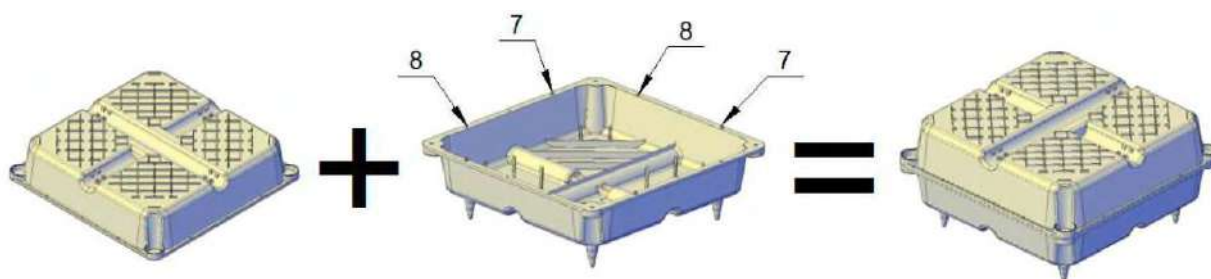
Рисунок 2. Общий вид пустотообразователя составной формы
