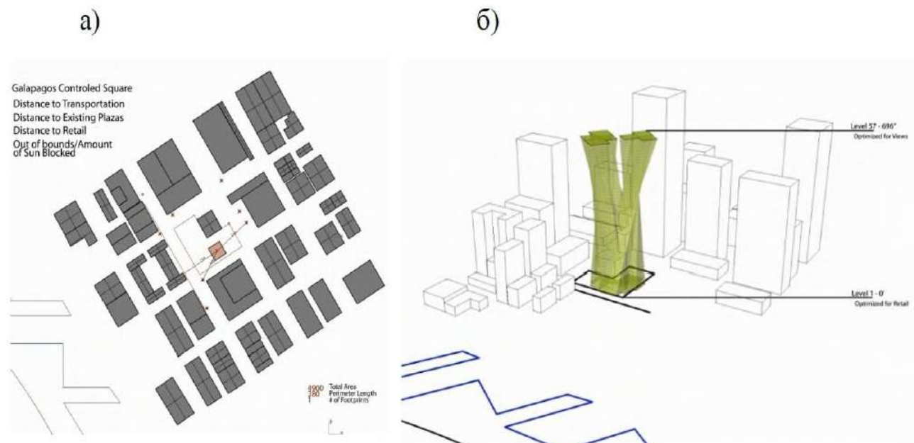
Рис.6. – Генерация формы в Galapagos: а) задание граничных условий; б) оптимальный вариант формы.
