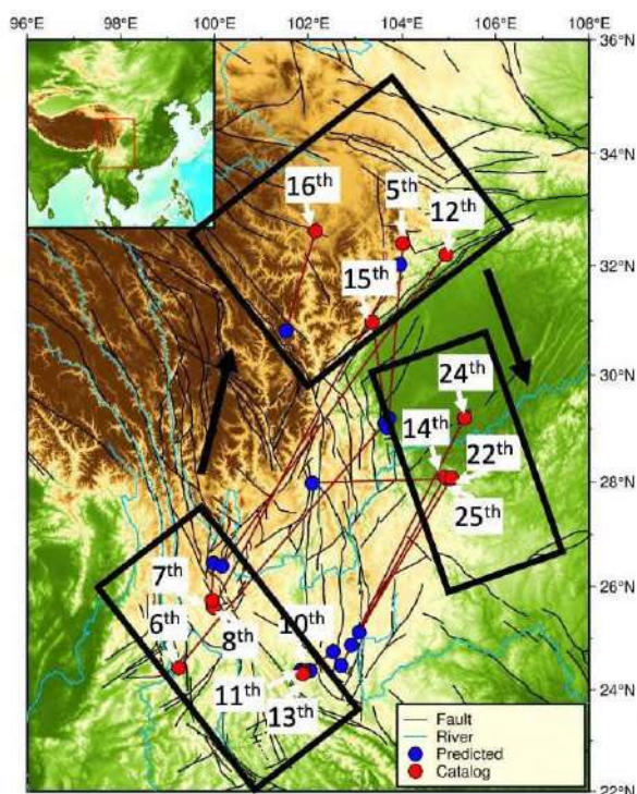
Рис 2. 1) разломы (чёрные линии), 2) реки (синие линии). Данные о землетрясениях: 3) красные круги - эпицентры ранее зафиксированных землетрясений. 4) синие круги - прогнозируемые эпицентры землетрясений на основе геологических моделей.
