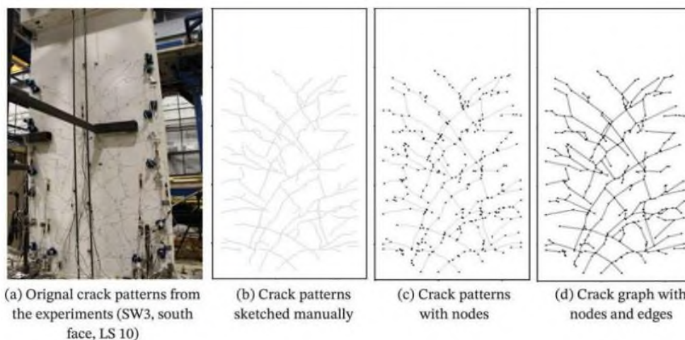
Рис.1(a) Оригинальные трещины из экспериментов (SW3, южная сторона, LS 10); (b) Шаблоны трещин, нарисованные вручную; (c) Шаблоны трещин с узлами; (d) Граф трещин с узлами и рёбрами.
