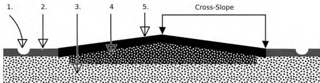
Сурет 2 Жолдың қимасы: 1. Дренаждық құбыр; 2. Көлік тоқтауға арналған бекет; 3,4-Жол қабаты; 5. Асфальт
