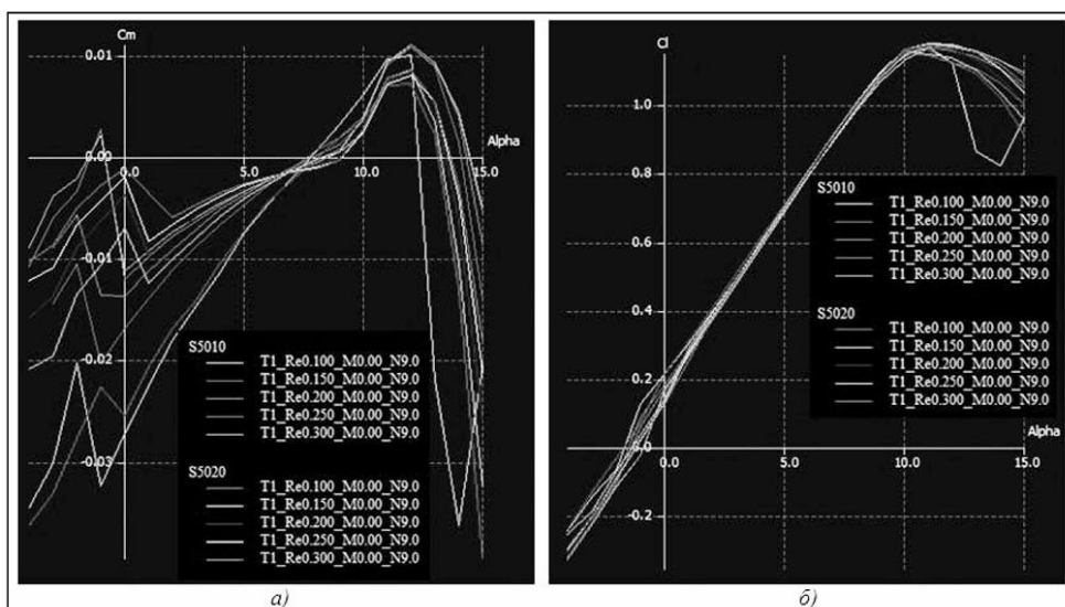
3-сурет. Көтергіш күш коэффициентінің шабуыл бұрышына тәуелділік графигі
