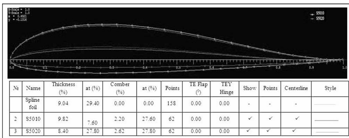
2-сурет. XFLR5 бағдарламасында есептелген S5010 және S5020 профильдерінің аэродинамикалық беттері
