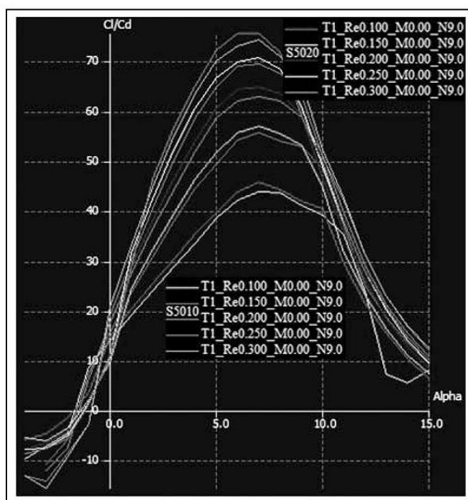
4-сурет. C_l/C_d коэффициентінің шабуыл бұрышына тәуелділік графигі
