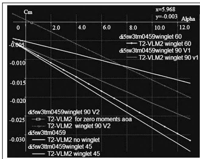
5-сурет. Күш моментінің шабуыл бұрышына тәуелділік графигі
