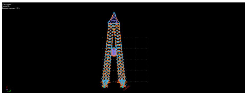
Рисунок 3 – эпюра крутящего момента M_z
