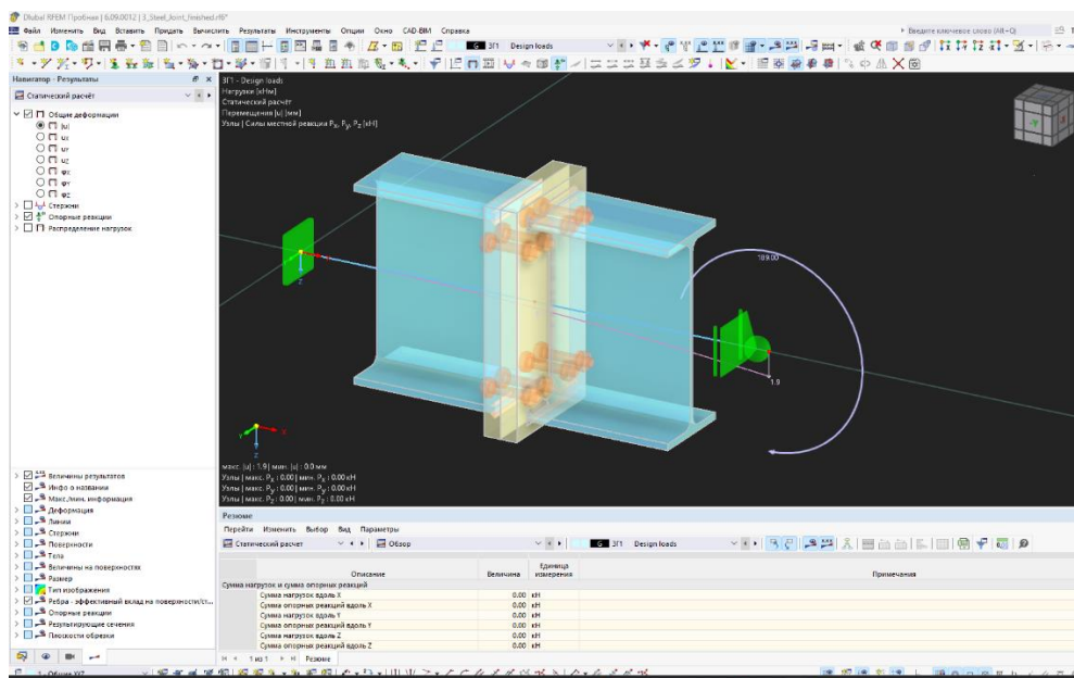
Рисунок 6 – деформация стального соединения
