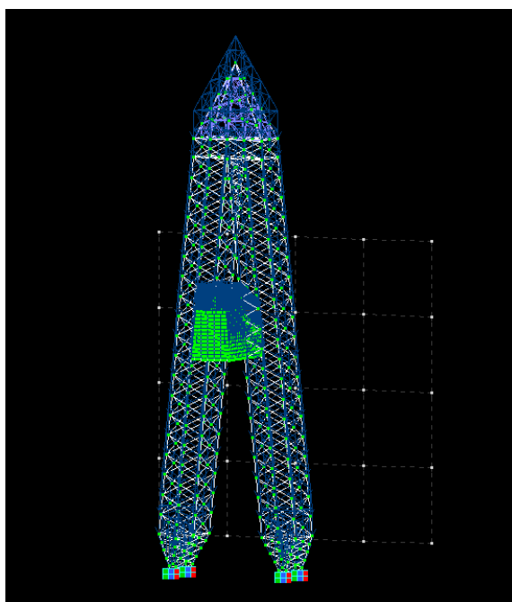
Рисунок 2 – наложения нагрузки собственного веса
