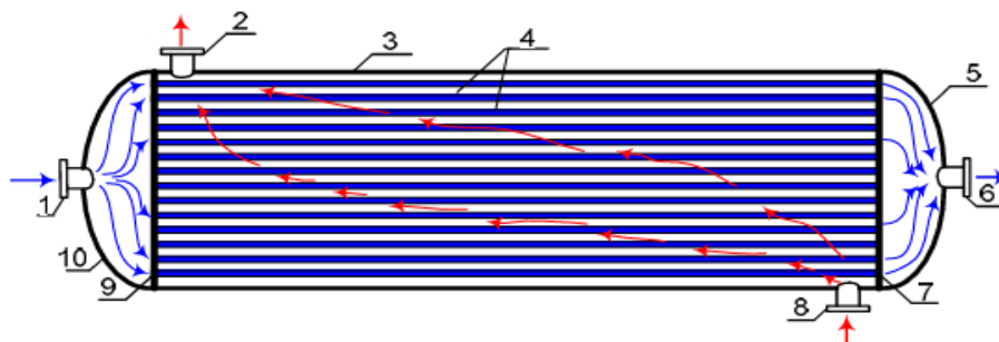
Сурет-1: Бірөтпелі қабықшатүтікшелі жылу алмастырғыштың құрылысы
