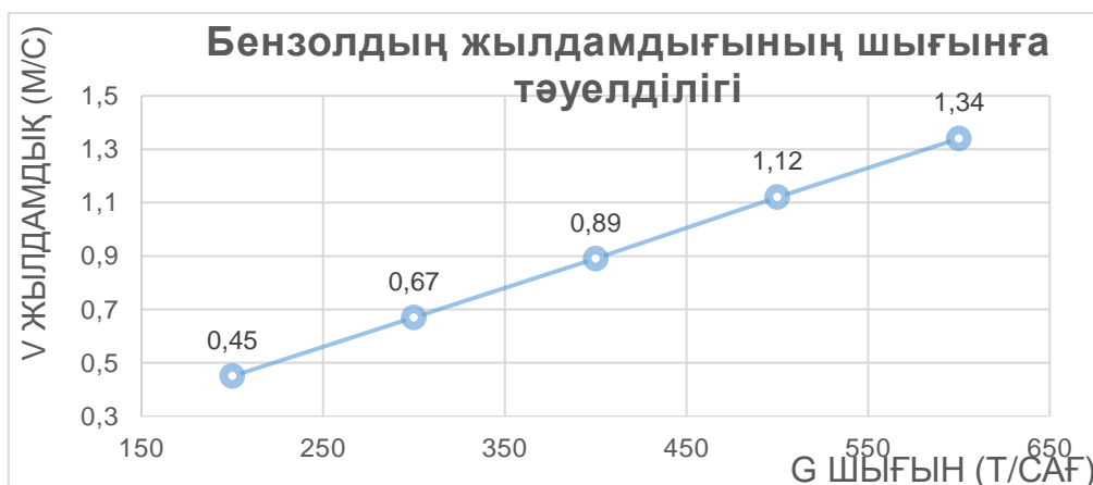
3-сурет: Бензолдың жылдамдығының шығынға тәуелділігі
