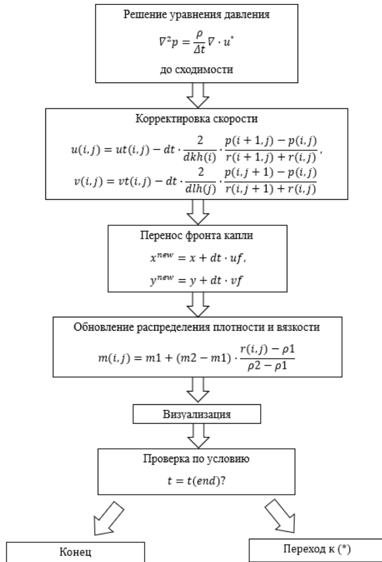
Рисунок 1 Алгоритм кода.
