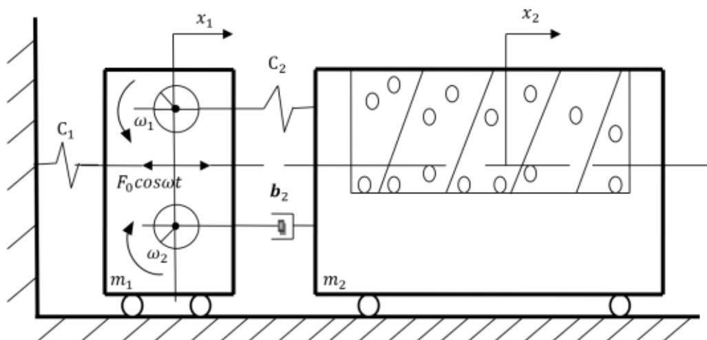
Рис. 1. Динамическая модель двухмассной горизонтальной площадки
