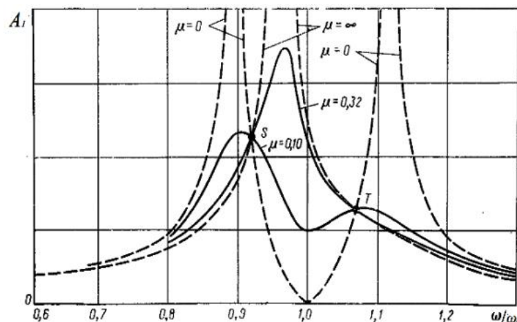
Рис. 2. Амплитудно-частотная характеристика двухмассовой машины с различной степенью диссипации
