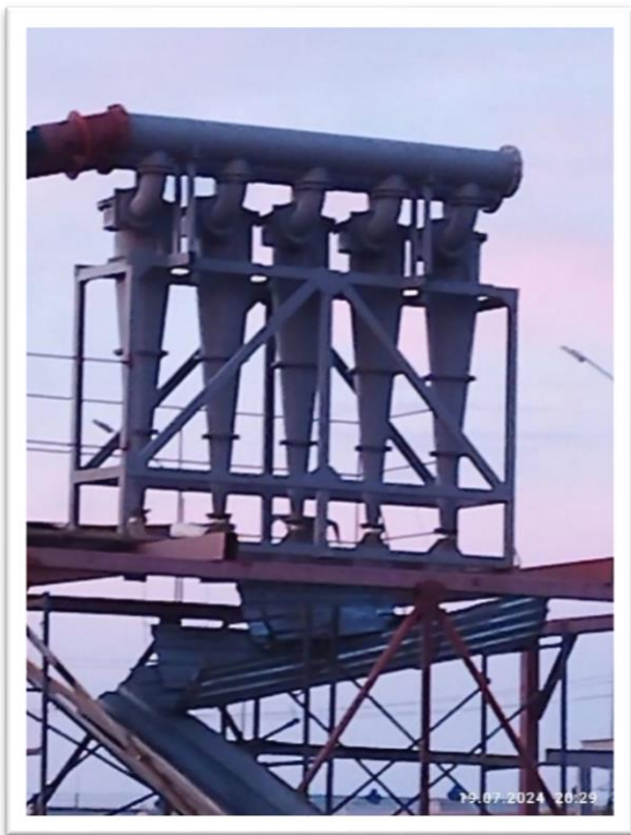
1-сурет. Өзен арнасын тазалауда гидроциклондарды қолдану
