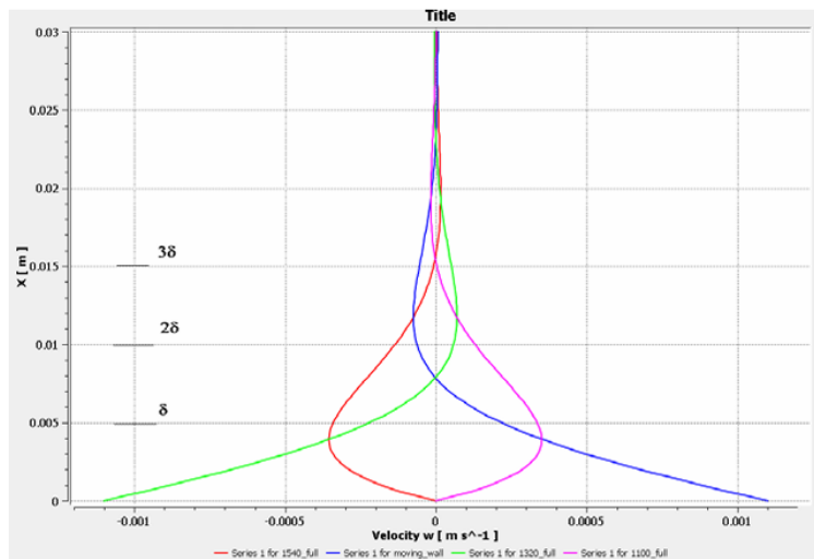
Рисунок 4. Распределение скорости, полученное численным анализом
