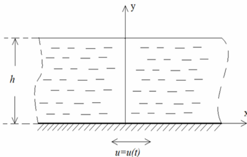
Рисунок 1. Область жидкости с подвижной стенкой
