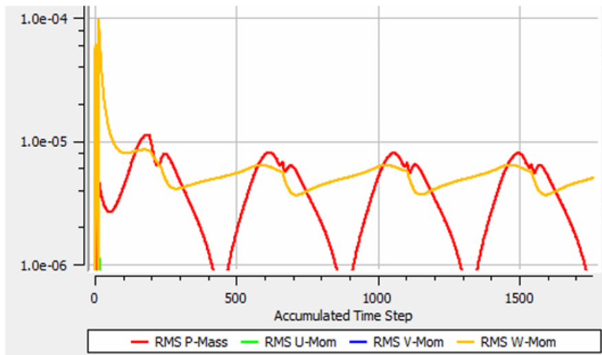
Рисунок 3. Изменение погрешностей вычислений при расчетах
