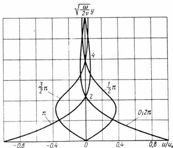
Рисунок 2. Профиль скорости у колебательной пластины
