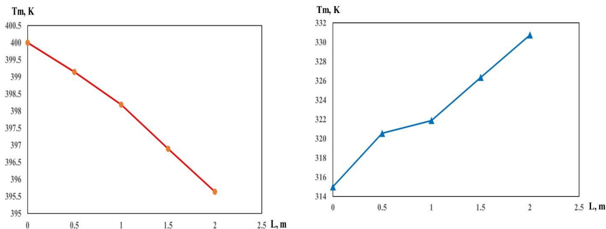
Рисунок 1. Распределение среднемассовой температуры нефти и воды вдоль ТОА (в первом граничном условии). Синяя линия — результаты для нефти, красная линия — результаты для воды.
