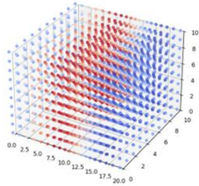
Сурет 2 Бойлық толқынның таралу көрінісі.
