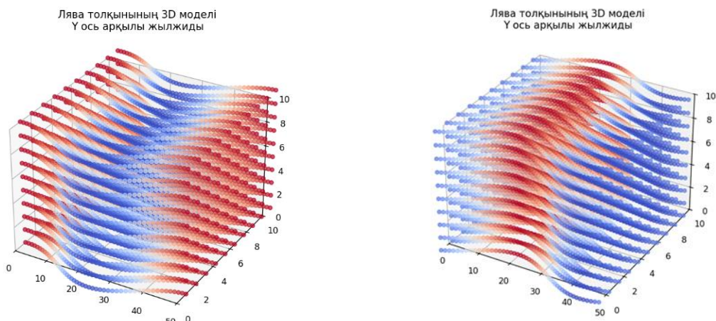
Сурет 5 Лява толқындардың таралу көрінісі.
