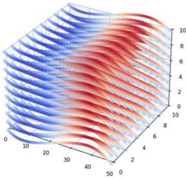
Көлденең толқынның 3D моделі(поперечная волна) Y ось арқылы жылжиды
