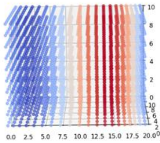
Сурет 2 Бойлық толқынның таралу көрінісі.
