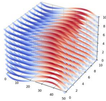
Сурет 3 Көлденең толқынның таралу көрінісі.
