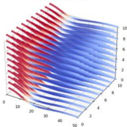
Рэлей толқынының 3D моделі Y, Z ось арқылы жылжиды
