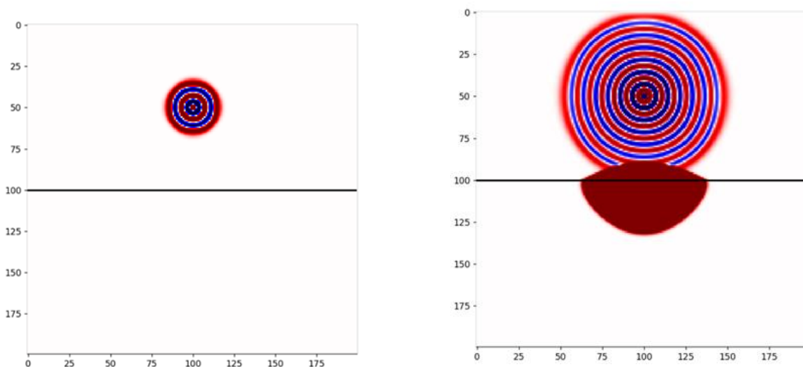
Сурет 6 Сфера түрінде таралатын толқындардың таралу көрінісі.
