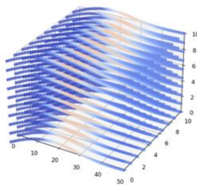
Сурет 4 Рэлей толқындардың таралу көрінісі.
