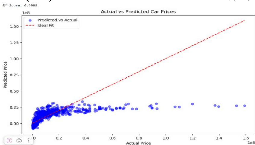
Рисунок 1. Применение линейной регрессии
