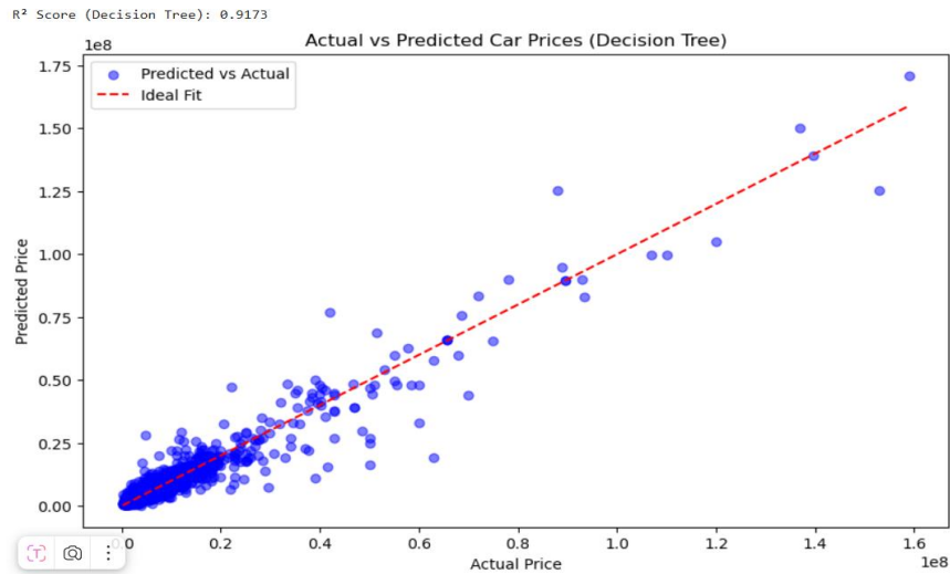
Рисунок 2. Применение метода дерева решений
