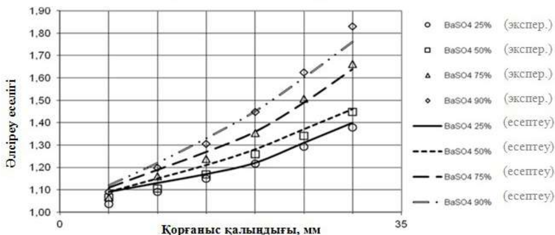
Сурет 2. BaSO 4 толтырғышы бар "Абрис Рзңқ-01" маркалы қорғаныс материалының қалыңдығына гамма-сәулелену дозасы қуатының әлсіреу еселігінің есептік және тәжірбелік тәуелділігі ( ^{198}\text{Au} көздері)
