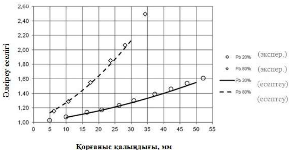
Сурет 3. Гамма-сәулелену дозасы қуатының әлсіреу еселігінің ( ^{60}\text{Co} көздері) Pb толтырғышы бар "Абрис Рзңқ-02" маркалы қорғаныс материалының қалыңдығына есептік және тәжірибелік тәуелділігі
