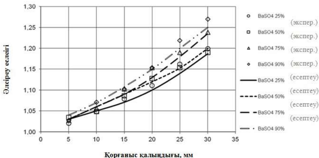
Сурет 1. BaSO 4 толтырғышы бар "Абрис Рзңқ-01" маркалы қорғаныс материалының қалыңдығына гамма-сәулелену дозасы қуатының әлсіреу еселігінің ( ^{60}\text{Co} көздері) есептік және тәжірбелік тәуелділігі.
