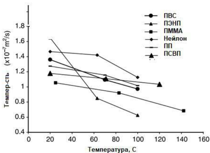
Рис 3. Температурная зависимость коэффициента температуропроводности образцов
