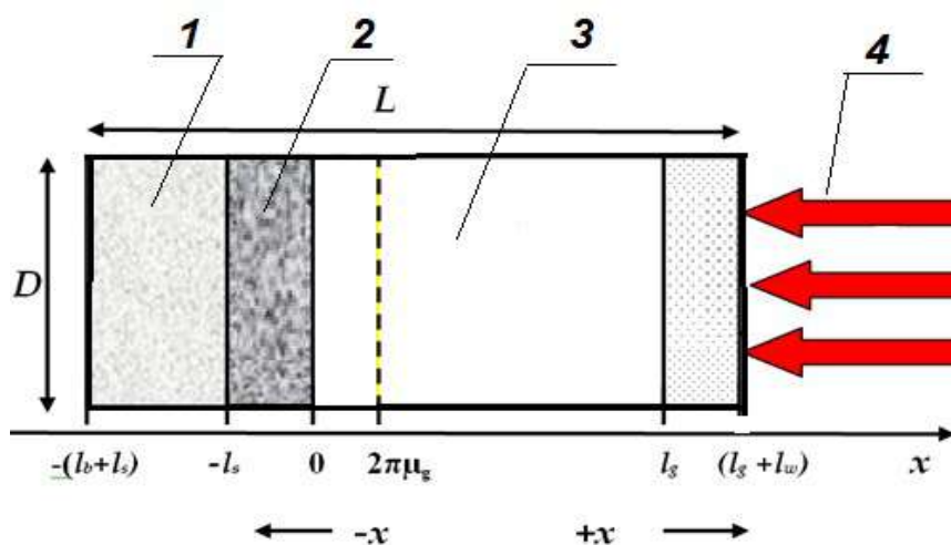
Рис.1. Поперечный разрез ФА камеры 1- положка;2- исследуемый образец; 3- газовый слой (воздух); 4- падающий модулированный лазерный луч, D–диаметр, L–длина ФА камеры.
