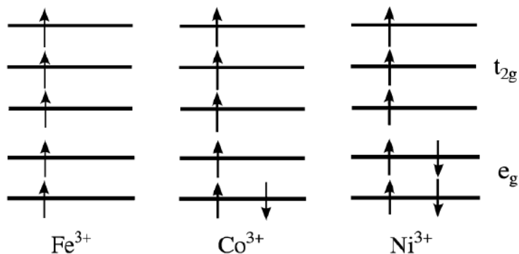
Рисунок 3. Схема, показывающая орбитальное заполнение 3d-электрона для примесей металлов в CuGaS2.
