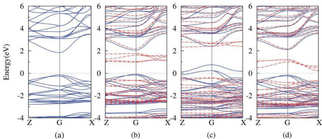
Рисунок 2. Спин-поляризованные зонные структуры чистого кристалла CuGaS2 (a) и кристалла CuGaS2, допированного Fe (b), Co (c), Ni (d). Сплошные (синие)/пунктирные (красные) линии обозначают спин вверх/вниз соответственно. Горизонтальная пунктирная линия обозначает уровень Ферми.
