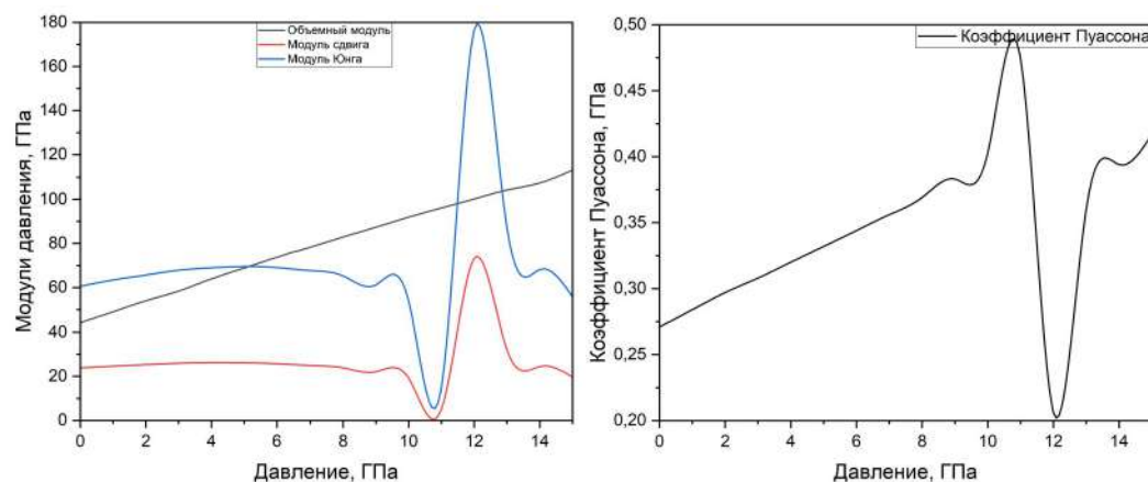
Рис.2. Изменение модулей упругости относительно приложенного гидростатического давления.
