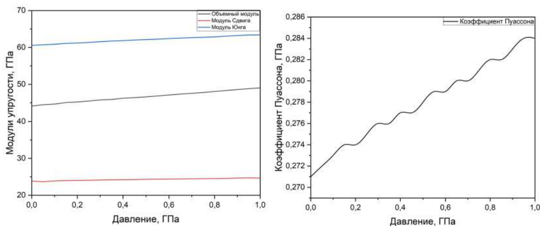
Рис.1. Изменение модулей упругости относительно приложенного гидростатического давления.
