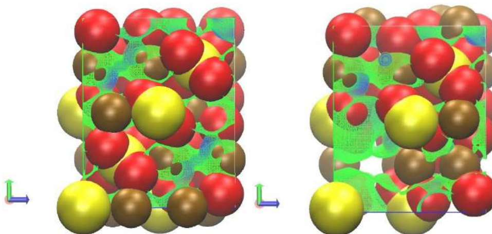
Рис.5. Карта электронной плотности, без дефекта (слева) и с дефектом (справа)
