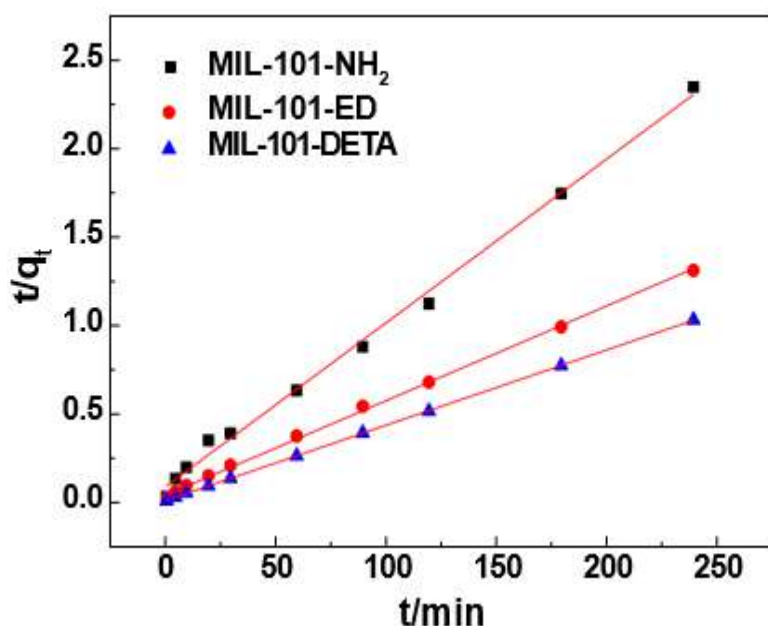
Сурет-1. MIL-101-NH 2 , MIL-101-ED және MIL-101-бөлшектеріндегі U (VI) сорбциясы үшін жалған бірінші ретті кинетикалық модель (жоғарғы) және жалған екінші ретті кинетикалық модель (төменгі) сызықтық аймақтары.
