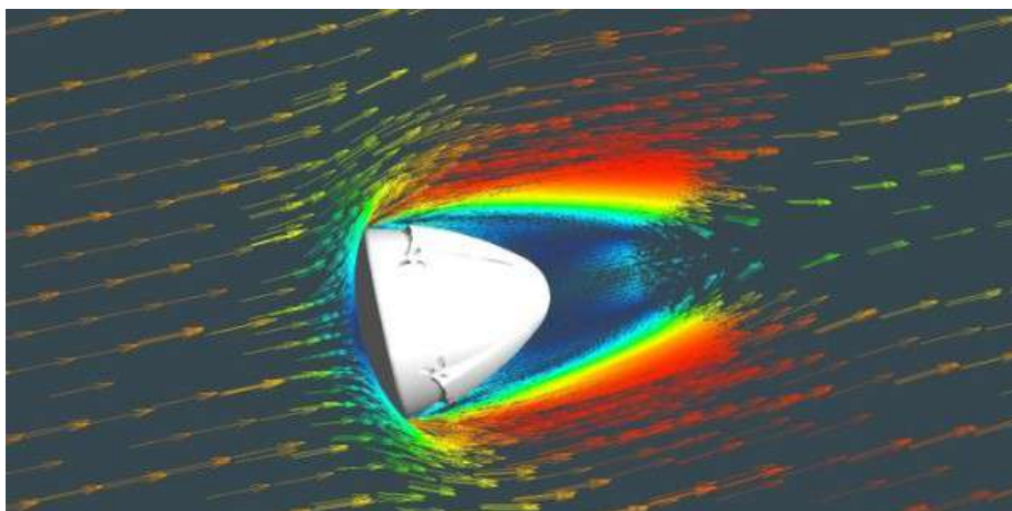
Рисунок 3 – Моделирование тепловых нагрузок на КА в программе ANSYS
