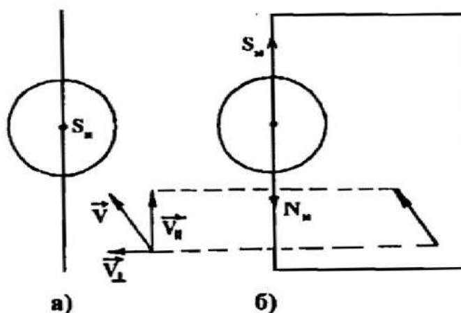
Сурет 1 - Бөлшектердің қозғалысын екі қозғалысқа бөлу: а – жоғарыдан көрініс; б – меридиан жазықтығындағы көрініс. [1, б.119]
