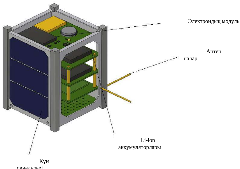
Сурет 1 - Дизайн элементтері мен құрамдас белгілермен модульдік CubeSat платформасының CAD моделі
