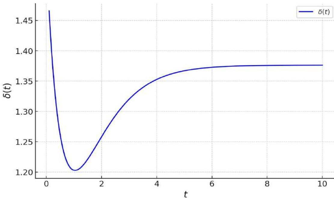
Сурет 1 – Жаңартылған гравитацияда материя тығыздық ұйытқуының эволюциясы
