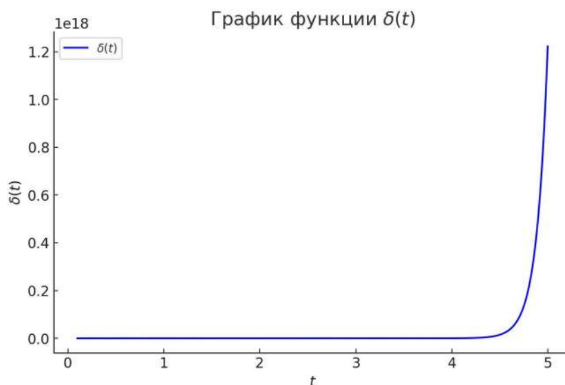
Сурет 1 - \delta(t) функциясының өзгерісі
