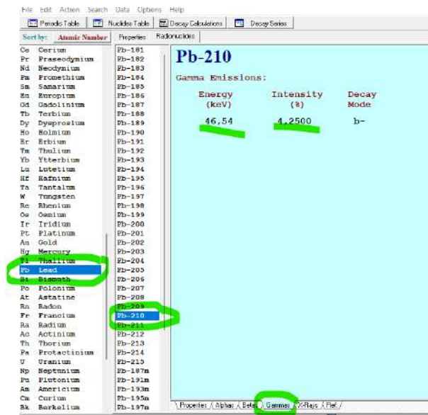
Сурет 4 – Қорғасын-210 ( ^{210}\text{Pb} ) изотопының гамма-сәулелену сипаттамасы
