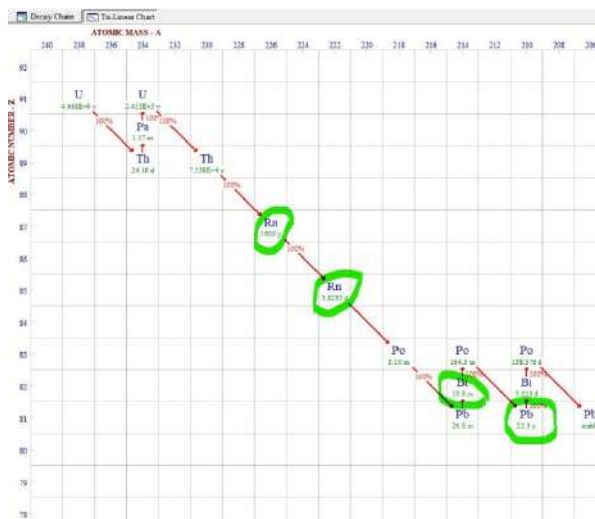
Сурет 2 - Уран-238 ( ^{238}\text{U} ) ыдырау тізбегі
