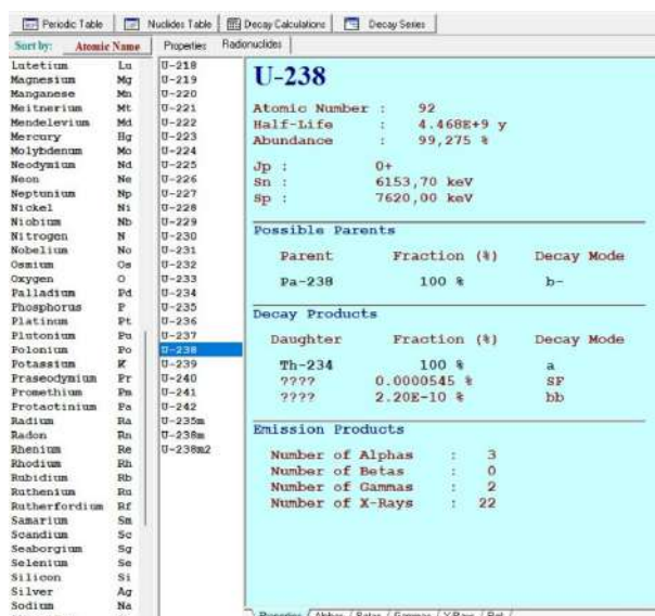
Сурет 1 – Уран-238 изотопының сипаттамасы және ыдырау өнімдері
