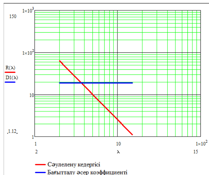
Сурет-1. Сәулелену кедергісі мен бағытталу әсер коэффициентінің толқын ұзындығына тәуелді графигі
