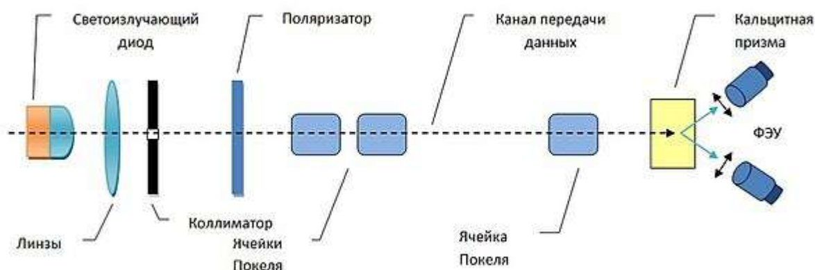
Сурет-2. Кванттық криптографияның BB84 хаттамасы.
