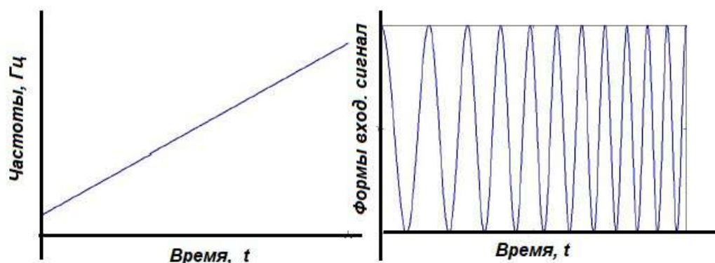
Рисунок 2. Линейная частотная модуляция сигнала
