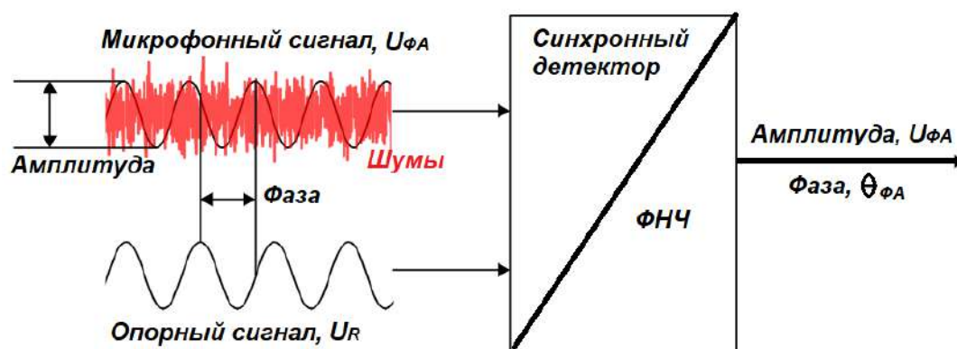
Рисунок 1. Принцип синхронного детектирования ФА сигнала
