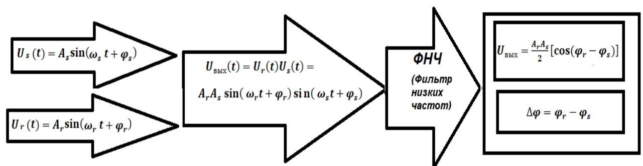
Рисунок 3. Схематичное представление синхронное детектирование ФА сигнала.
