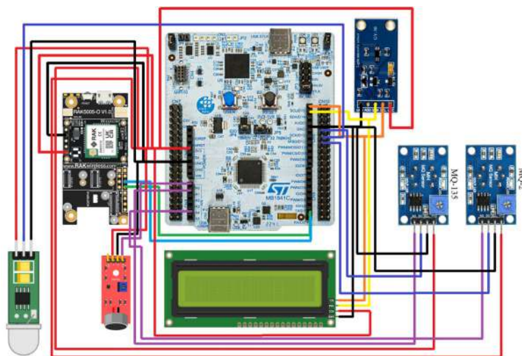
Рисунок 1. Схема стенда
