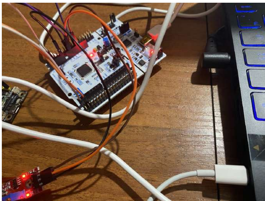
Рисунок 5. Подключение платы к компьютеру
