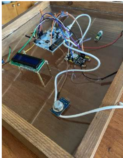
Рисунок 2. Физическая реализация стенда
