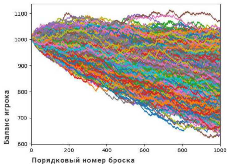
Рисунок 1. Моделирование Монте-Карло
