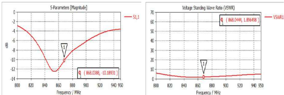
Рисунок 3. Результаты моделирования печатного диполя на частоте 868 МГц (S 11 параметр и КСВ)
