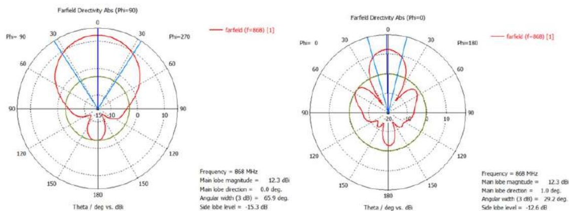
Рис. 3 — Диаграмма направленности при \varphi = 90^\circ и \varphi = 0^\circ
