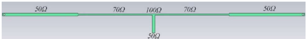
Рис. 2 Распределение сопротивление на геометрии антенны
