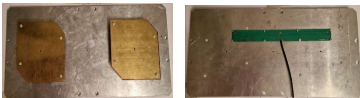
Рисунок 4. Внешний вид разработанной антенны в сборе
