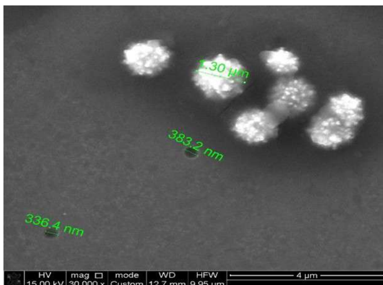
Рисунок 1 СЭМ изображение поверхности образца CuO / SiO 2 / Si после электрохимического осаждения при напряжении 2.5 В
