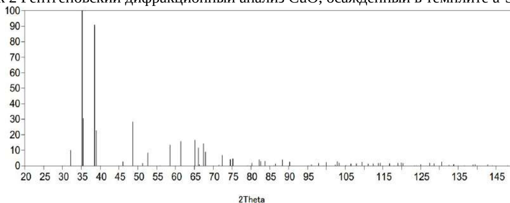
Рисунок 2 Рентгеновский дифракционный анализ CuO, осажденный в темплите \alpha -SiO 2 /Si-n
