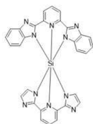
Si-hetero-1 Si(bzimpy/IPI)
