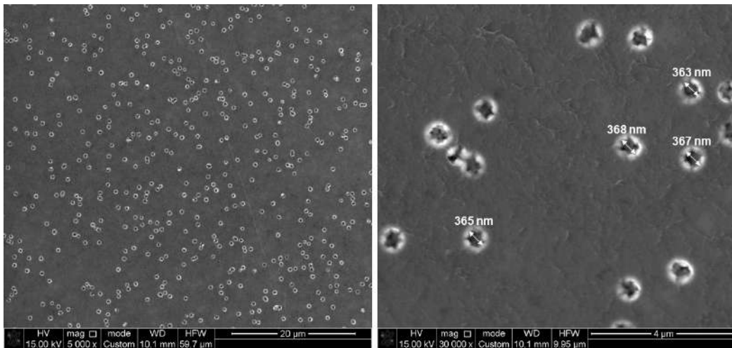
2-сурет. 30 минут аралығында өткен химиялық тұндырудан кейінгі беттің СЭМ кескіні.
