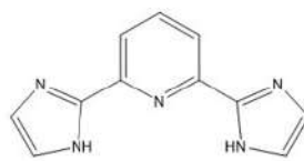
IPI - L2
