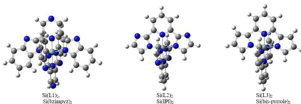
Рисунок 3. Оптимизированные структуры гомолептических соединений
