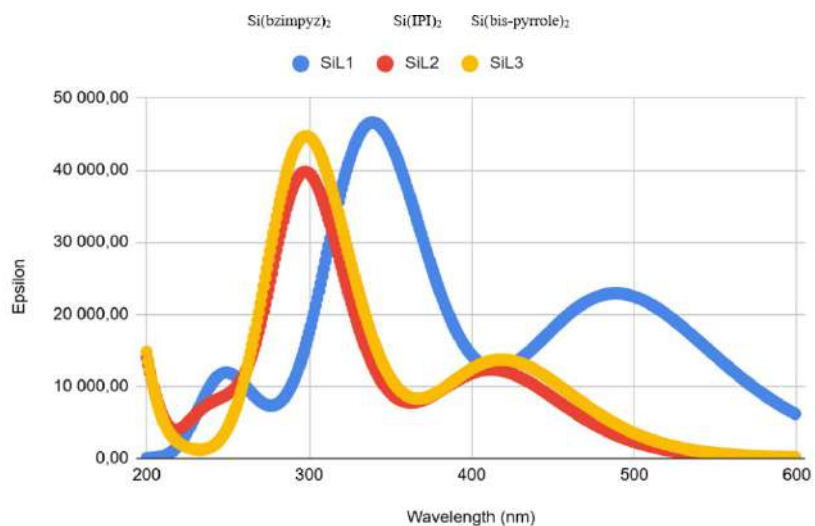
Рисунок 5. UV-Vis спектры гомолептических соединений
