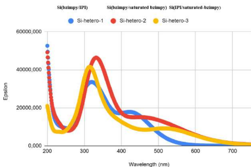
Рисунок 6. UV-Vis спектры гетеролептических соединений
