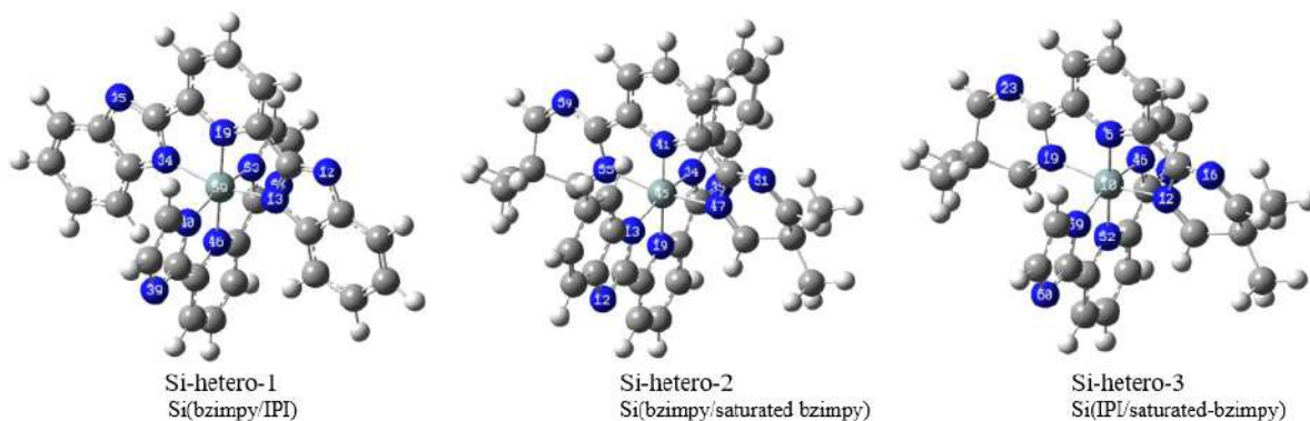
Рисунок 4. Оптимизированные структуры гетеролептических соединений
