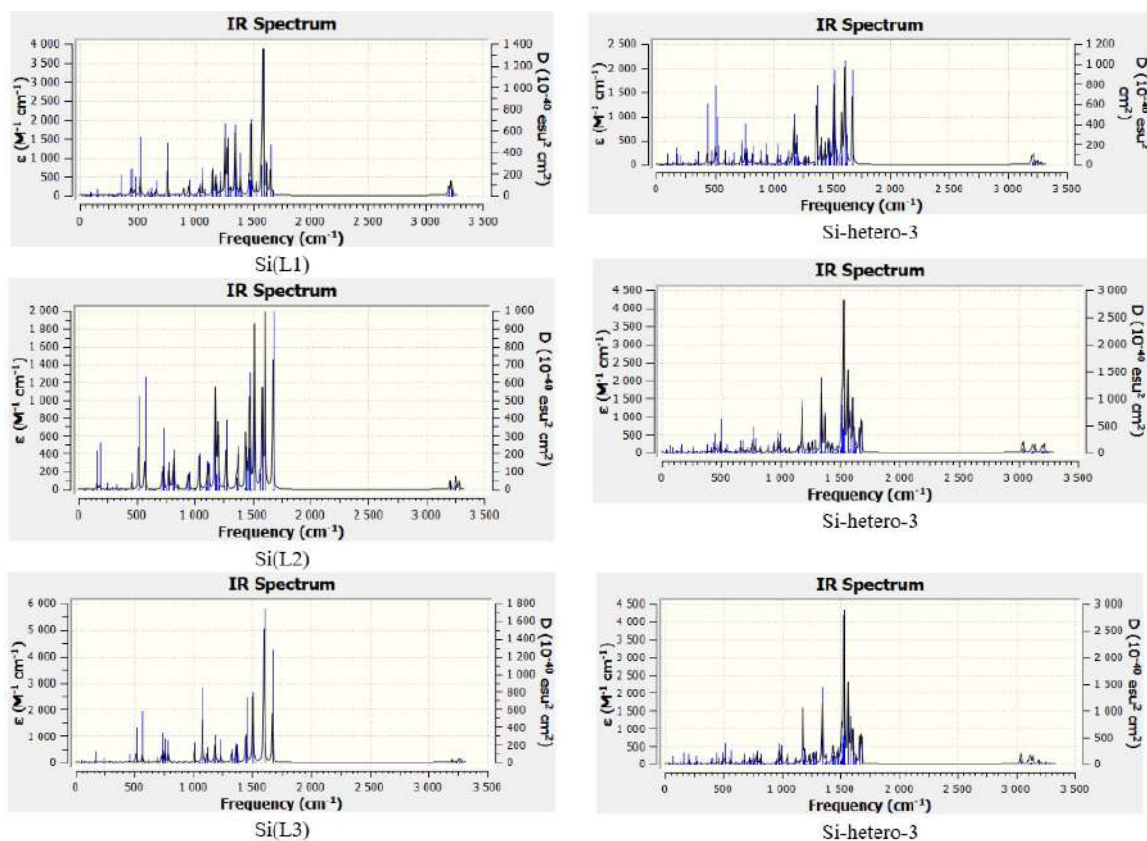
Рисунок 7. IR спектры гомолептических и гетеролептических соединений.
