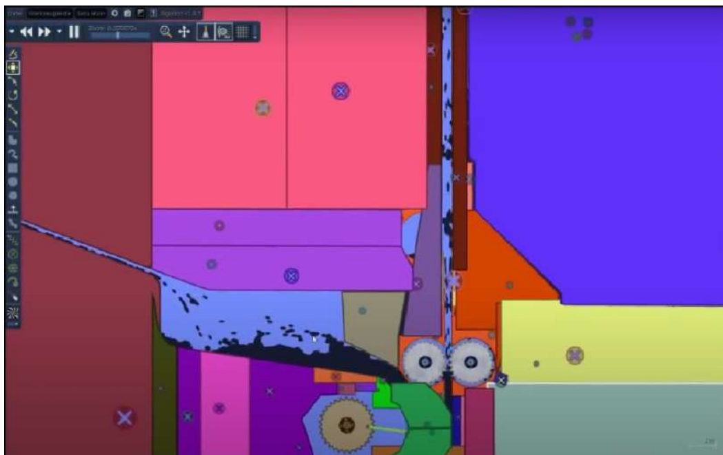
3 – сурет. Algodoo сайтында гидравликалық машинаның симуляциясы.
