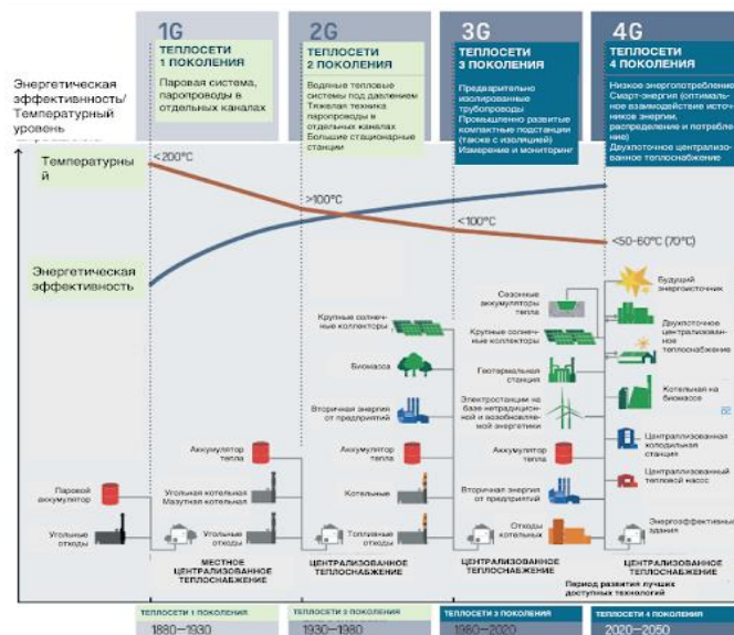
Рисунок 1 – Классификация систем теплоснабжения
