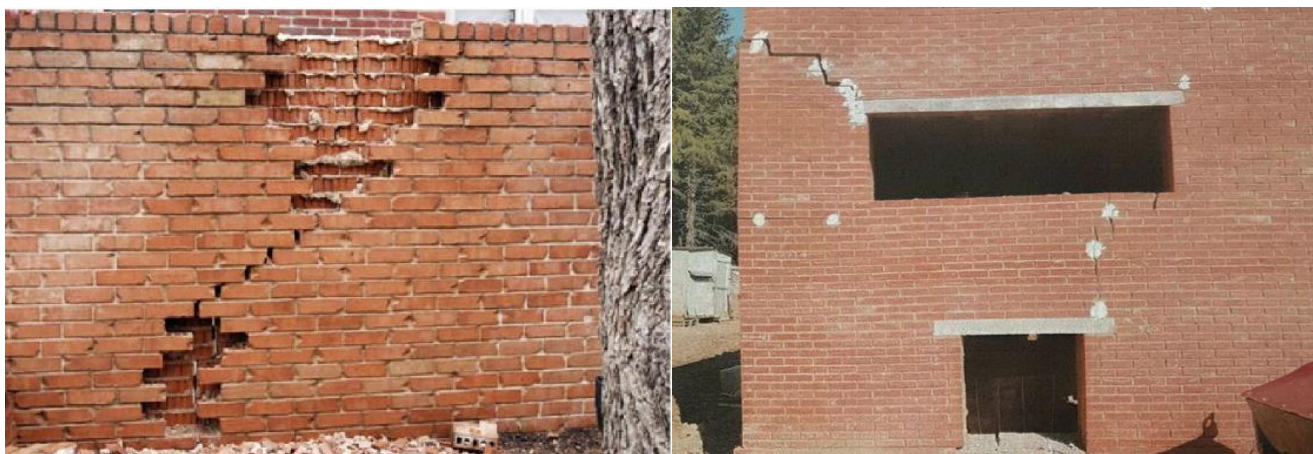
Рисунок 2. Расслоение кладки и выпадение отдельных камней, образование трещин.
