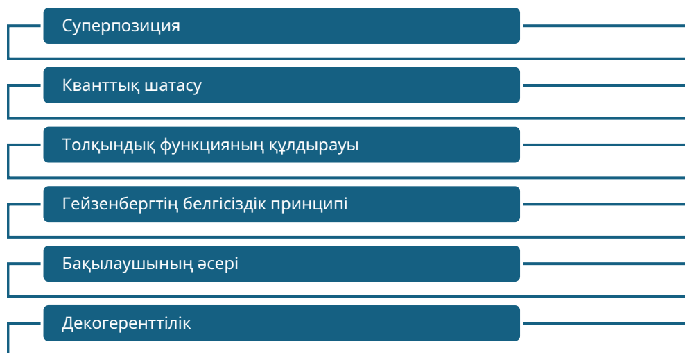
1-сурет. Сананың кванттық механика тұрғысынан түсіндіруде кванттық физикадан алынған принциптер
