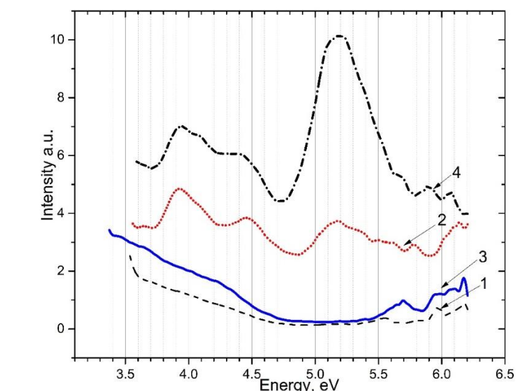
Сурет 2 – 2,9-3,1 эВ кезіндегі \text{CaSO}_4 -дің қозу спектрлері
