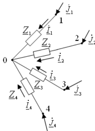
1 сурет – Радиал тізбектің схемасы
