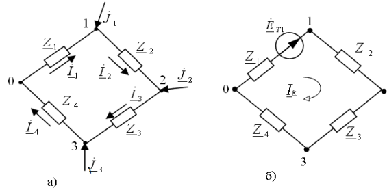
3 сурет – Түйықталған тізбектің схемасы а) бастапқы схемасы, б) есептік схемасы
