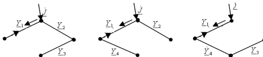
5 сурет – \underline{C}_{11} алымының бағытталған граф ағаштары
