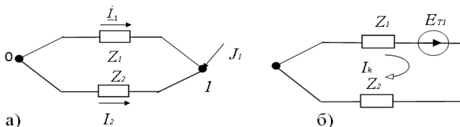
2-сурет – а) бастапқы схема; б) есептік схема
