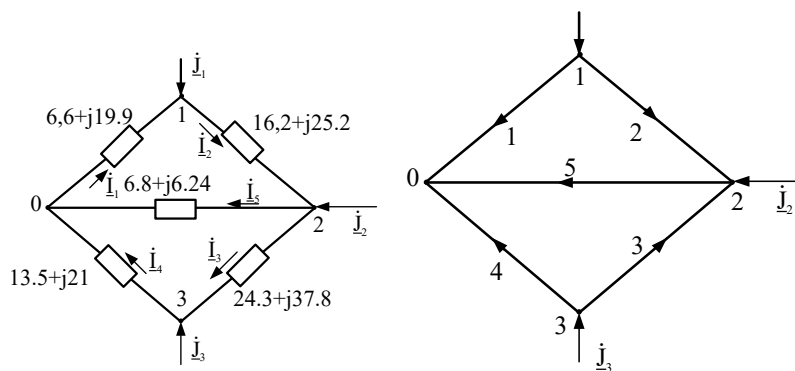
Рисунок 1 - Расчетная схема и направленный граф сети 110 кВ
