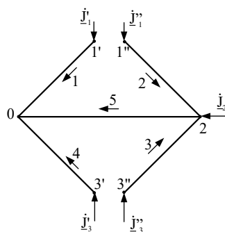
Рисунок 2 - Граф разомкнутых подсхем (') и (")
