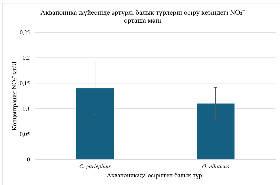
Сурет 2 Аквапоника жүйесінде әртүрлі балық түрлерін өсіру кезіндегі NO 2 - орташа мәні
