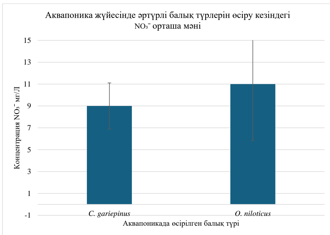
Сурет 4 Аквапоника жүйесінде әртүрлі балық түрлерін өсіру кезіндегі NO 3 - орташа мәні
