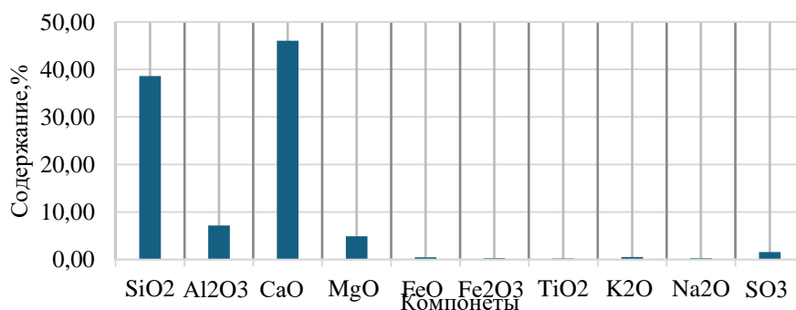
Рисунок 1 Химический состав образцов доменного шлака
