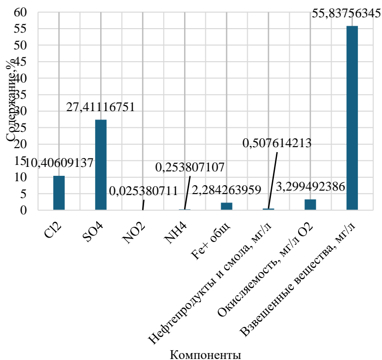
Рисунок 2 Химический состав сточных вод доменного шлака
