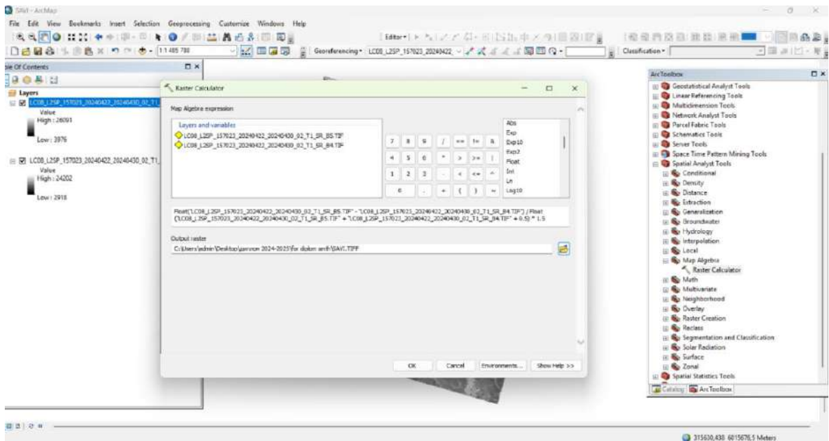
Сурет 3 SAVI индексін анықтау барысы
