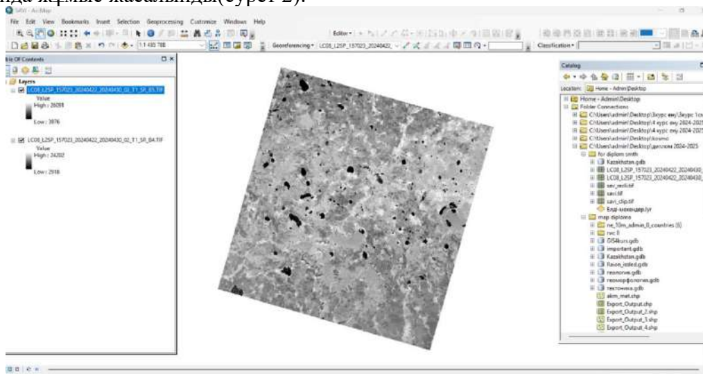
Сурет 2 ArcMap қосымшасына енгізілген 4, 5 каналдар
