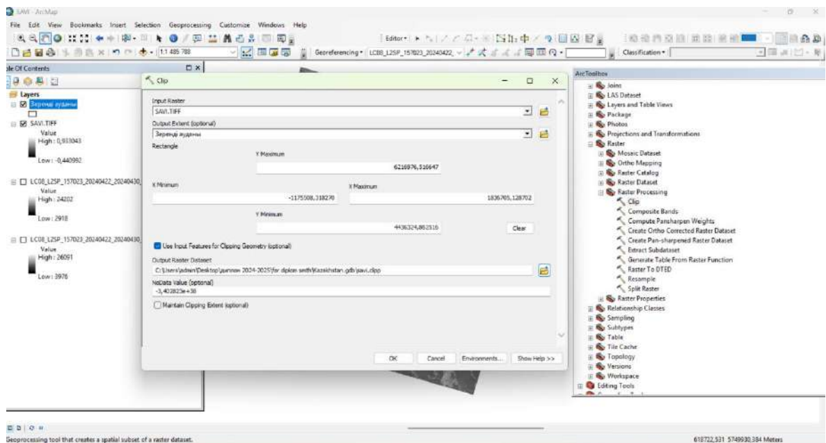
Сурет 4 Сіріп құралы көмегімен Зеренді ауданын кесіп алу
